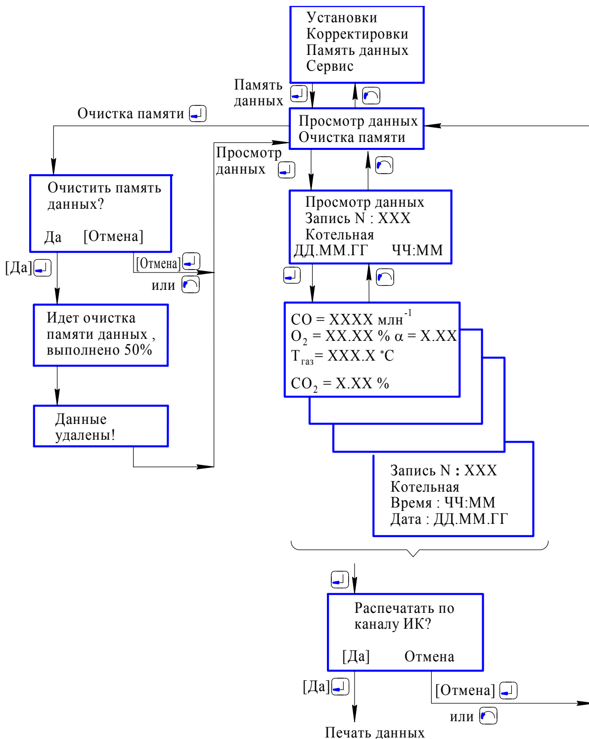
Рисунок 2.13 – Схема режимов работы газоанализаторов при печати по инфракрасному каналу связи и просмотра памяти данных
