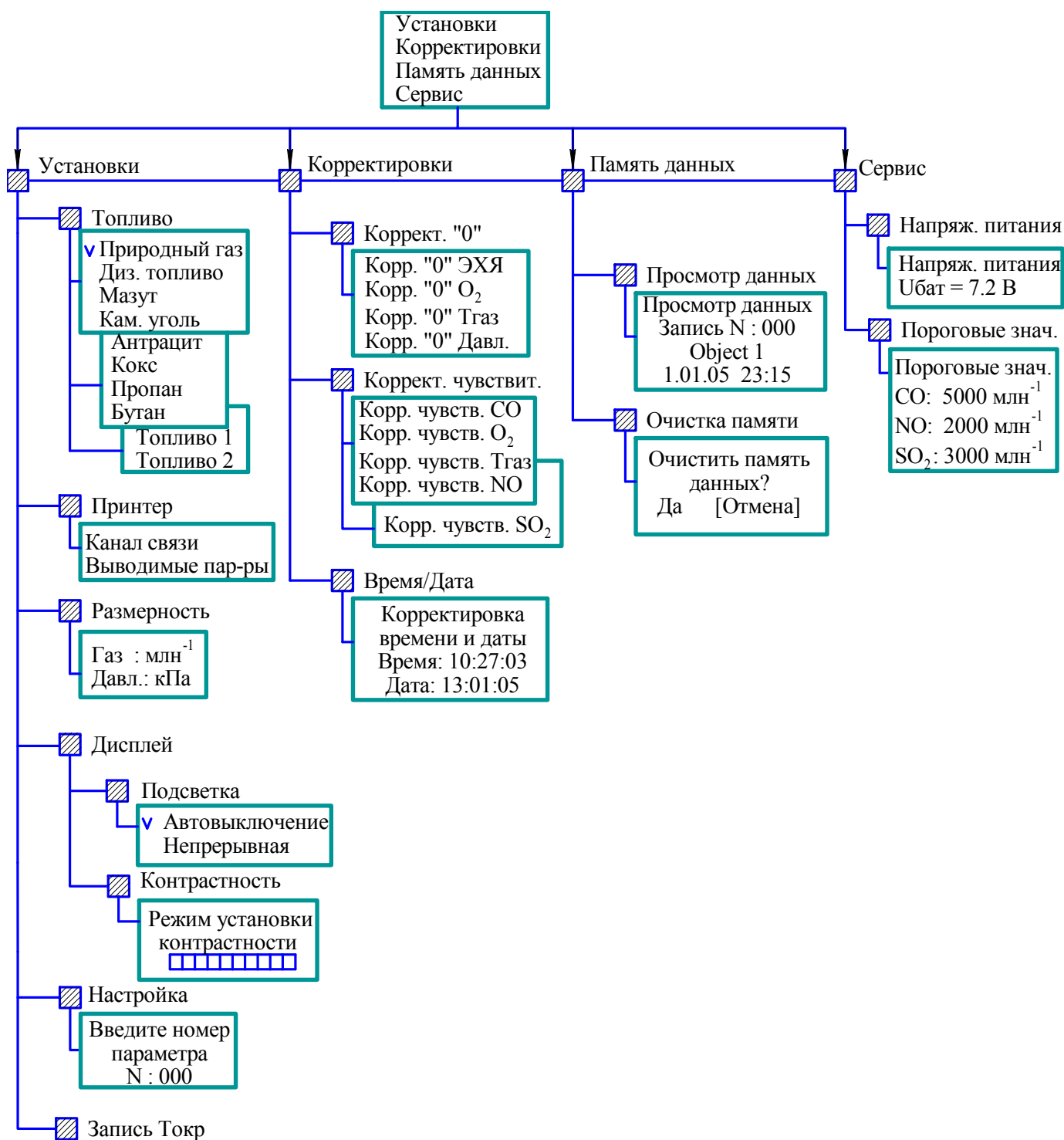
Рисунок 1.2 – Схема режимов работы газоанализаторов АНКAT-310
